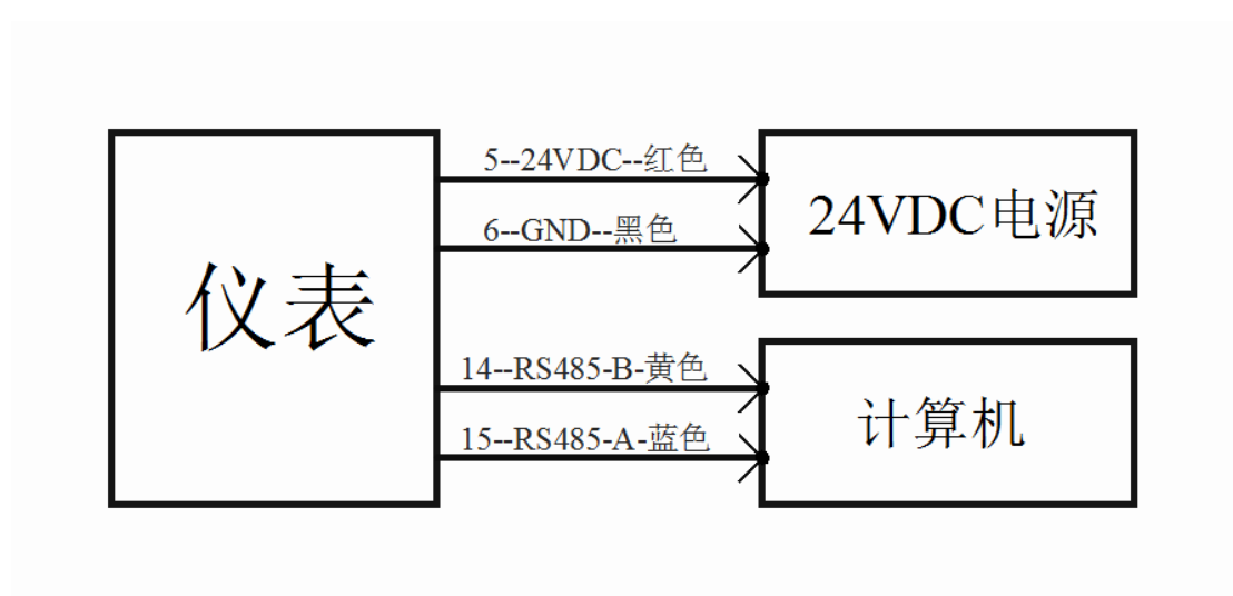
图一、仪表接线示意图
