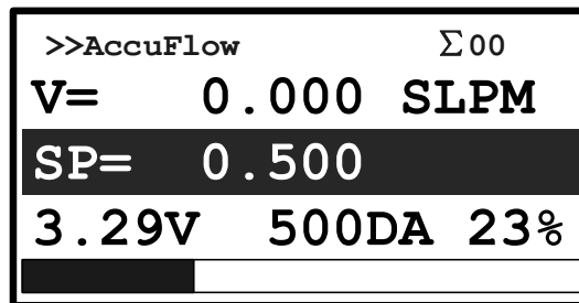
图2 阀控设定状态
