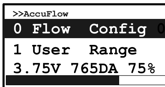
图2 阀控设定状态
